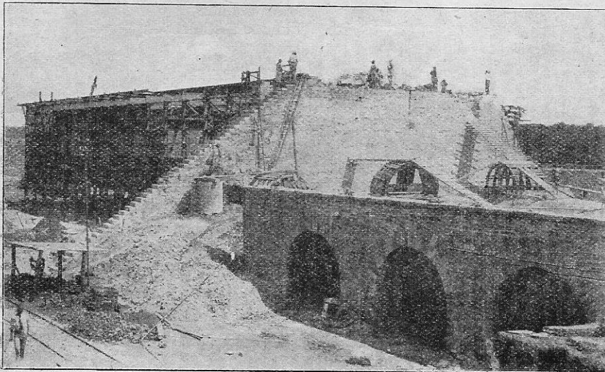
INSTELLINGEN IN OPBOUW VOOR HET AFLOSSEN VAN KOPERERTS IN KATANGA
